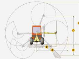
PRACOVNÍ ZÁBER
